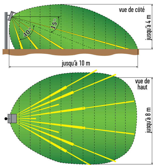
La zone de détection de la barrière MIR-M10
